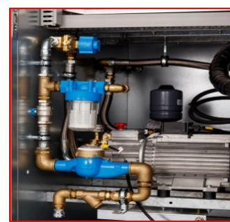
Maskinrum
